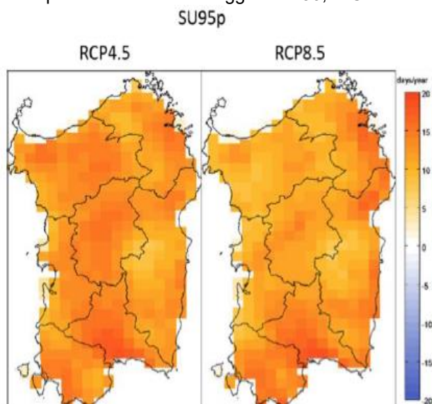
Figura 3-4: Anomalie (days/year, ossia giorni/anno) dell'indicatore SU95p riferito al numero medio di giorni all'anno con temperatura massima giornaliera maggiore di 30,1°C (SU95p) per il periodo 2021-2050 rispetto al periodo di riferimento 1981-2010 secondo gli scenari RC4.5 e RC8.5
